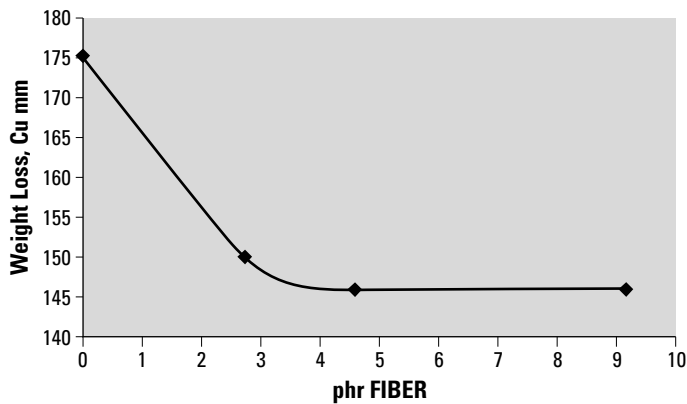
DIN Abrasion
